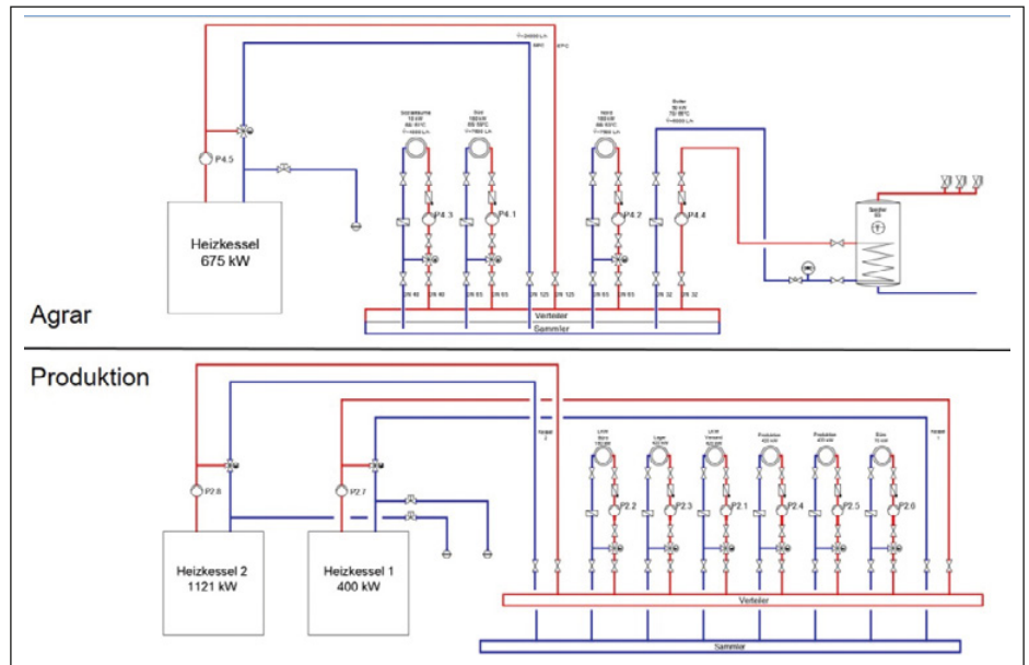
Grafik 1: Das alte Anlagenschema vor der Modernisierung bei Agrar und Produktion beim 70.000 m 2 großen Areal bei Dehner in Rain am Lech.
