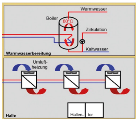
Grafik 4: Nutzung der Heizenergie.
